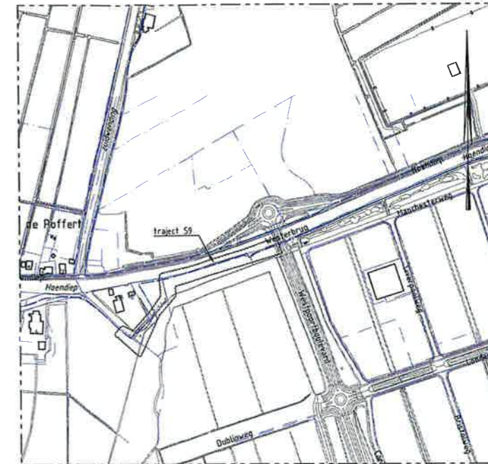
Overzicht schaal 1 : 5000
